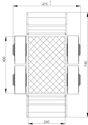
JFB 60 H | Art.No. 10 601 206-H| Draufsicht | Top view
