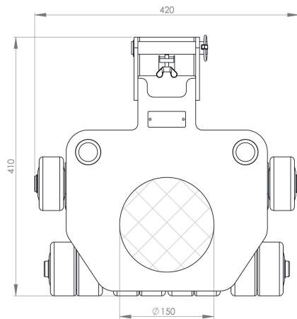
JLF 5 | Art-No. 16 050 085-D | Draufsicht | Top view
