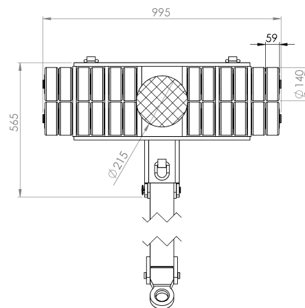
JLB 30 G | Art-No. 09 303 140-V | Draufsicht | Top view
