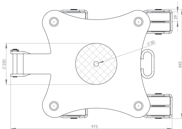
JKB 10 G | Art.No. 14 101 140-VU | Draufsicht | Top view
