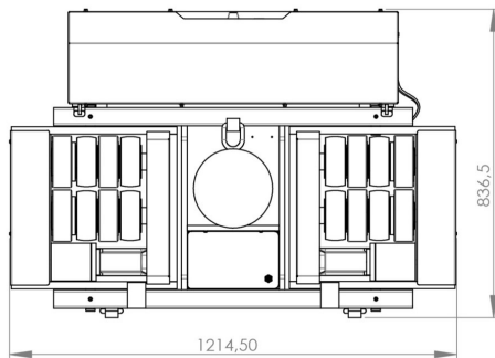
JLA-e 15/30 G | Art.No. 22 015 200-G| Draufsicht | Top view
