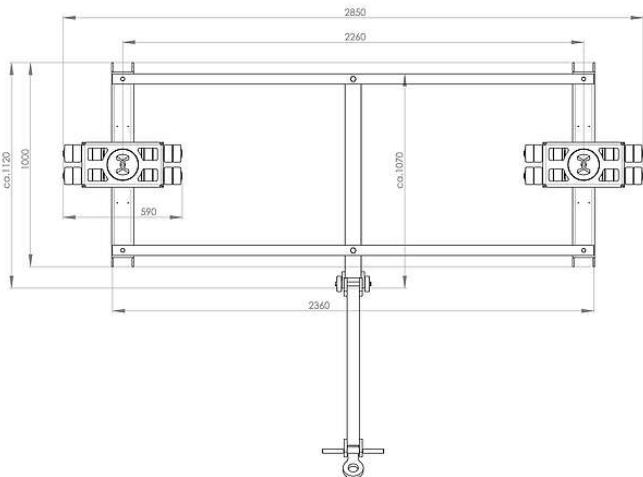
JTLB 14 K | Bestell-Nr. 12 121 085-WZ | Draufsicht JTLB 14 K | Order No. 12 121 085-WZ | Top view
