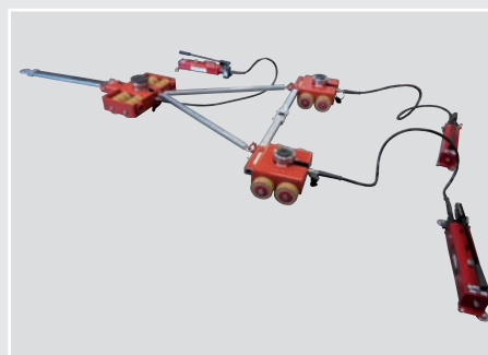
Chariot JLB 15 G et JFB 15 G avec levage intégré
