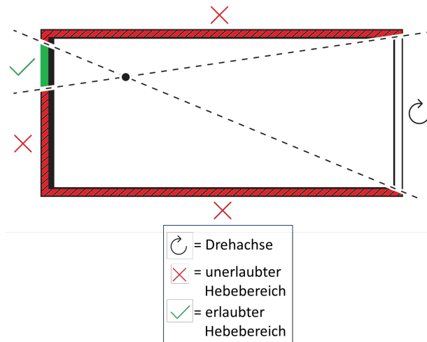
Abbildung 1 – Beispiel für die Ermittlung des erlaubten Hebebereichs
