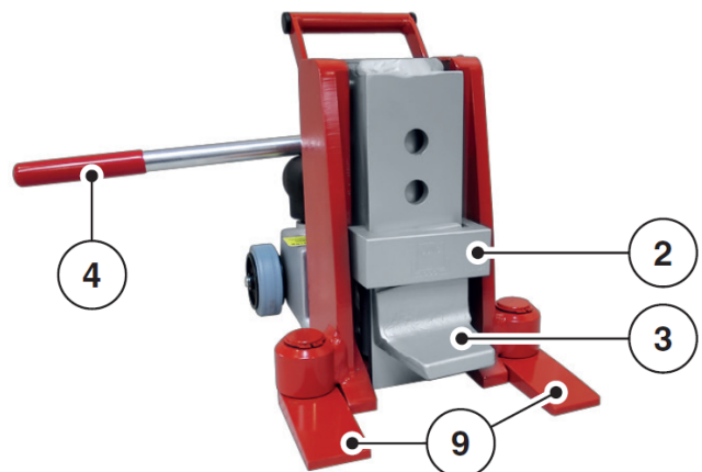
Abbildung 2 – Darstellung eines Hydraulikhebers mit Handhebelbedienung bestehende aus Lasche (3), Bügel (2), Pumpenhebel (4) und Schwenkfüßen (9)
